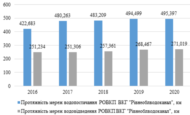
Рис. Протяжність мереж РОВКП ВКГ «Рівнеоблводоканал» у м. Рівне
