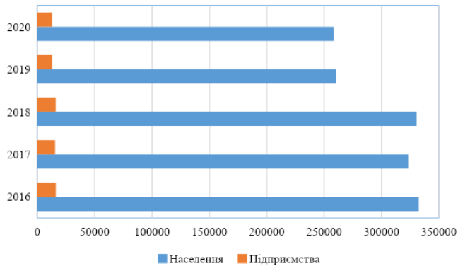
Рис. Споживання теплопостачання, Гкал
