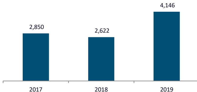
Рис. 14. Викиди забруднюючих речовин стаціонарними джерелами в атмосферне повітря (смт Квасилів і м.Рівне)
